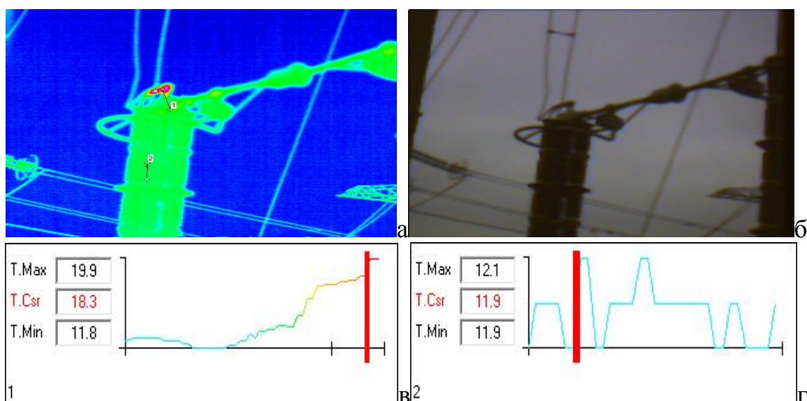
а) термограмма, б) оптический диапазон, в) график температур по сечению 1, г) график температур по сечению 2
