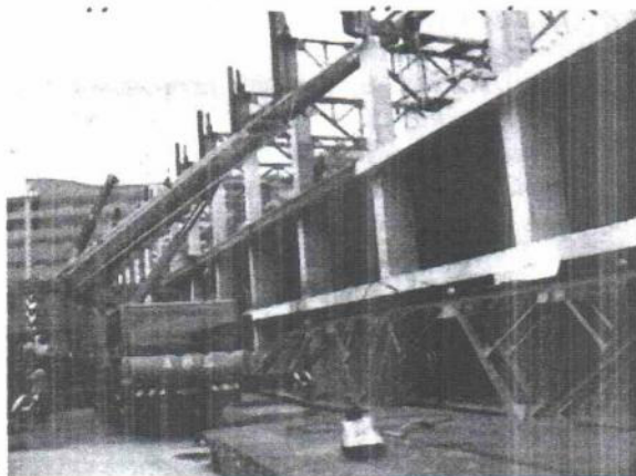
Рис. 2 Реконструкция промышленного здания (демонтаж плит покрытий) / Reconstruction of industrial buildings (dismantling of covering plates)
