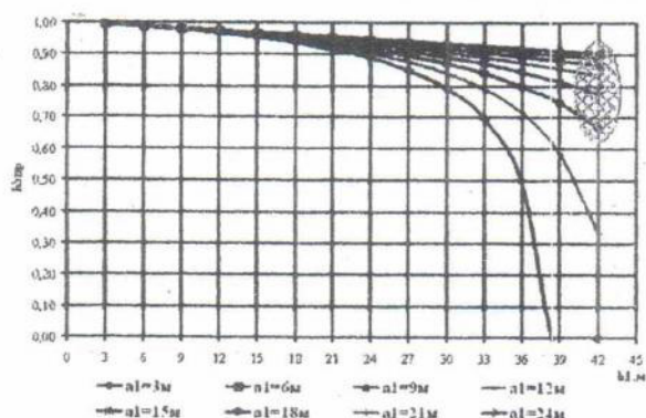
Рис. 3 Показатель безопасной организации зоны производства работ (при схемах организации зоны производства работ № 4) / Index of safe organization of execution area production of works (schemes of the organization of the area production of works № 4)
