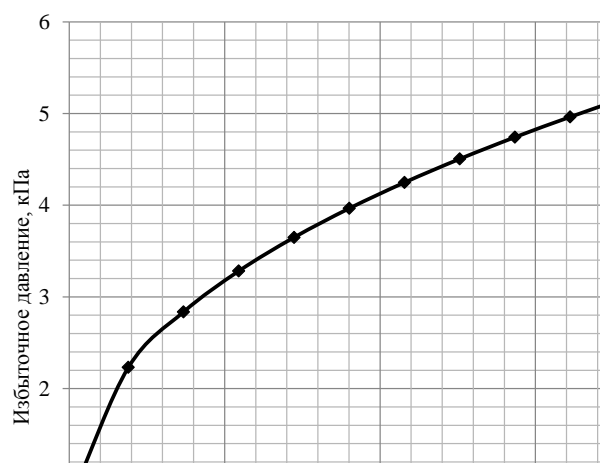
Рис. 5 – Избыточное давление в зависимости от коэффициента Z
