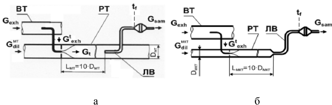
Рис. 2. Схемы минитоннеля (а) та микро-тоннеля (б) [5].
