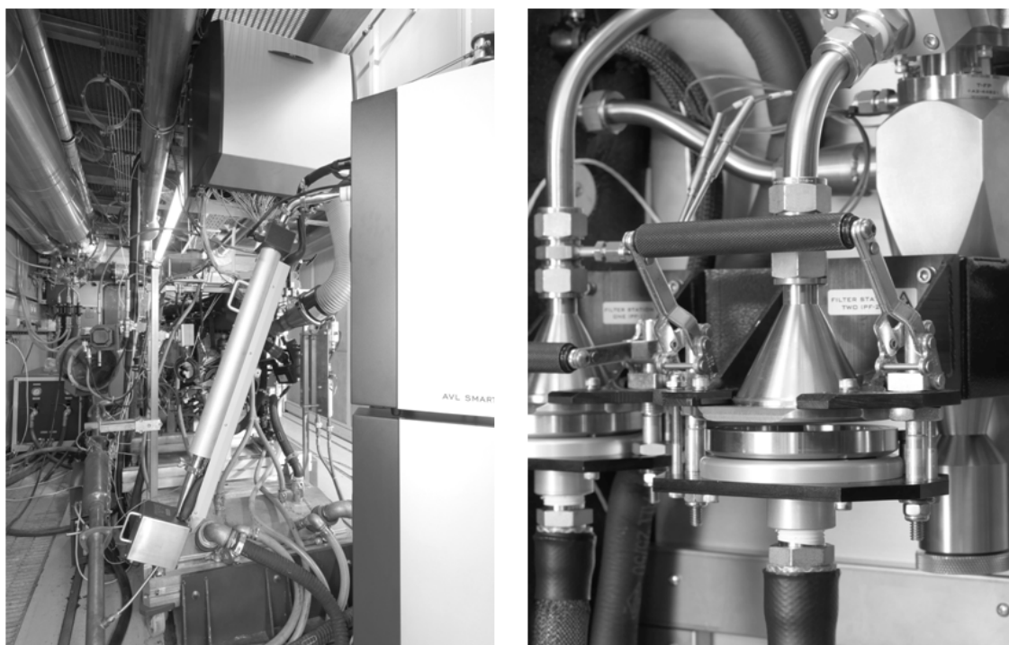
Рис. 4. Внешний вид частичнопоточного туннеля компании AVL (а) и его держателя фильтров (б) [7].
