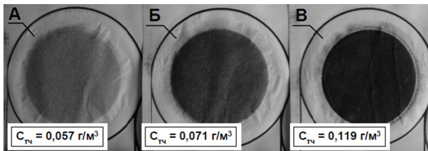
Рис. 3. Внешний вид тефлоновых фильтров, используемых в исследовании массового выброса ТЧ с потоком ОГ, стабилизированы и взвешены [6].
