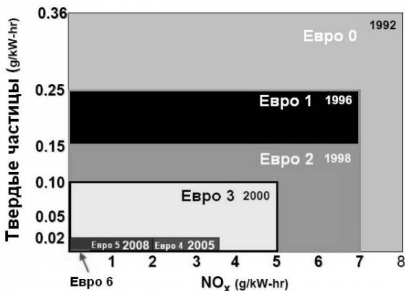
Рис. 1. Законодательно установленные требования экологическим показателям дизелей, в частности среднеэксплуатационные массовые выбросы оксидов азота и ТЧ [3].
