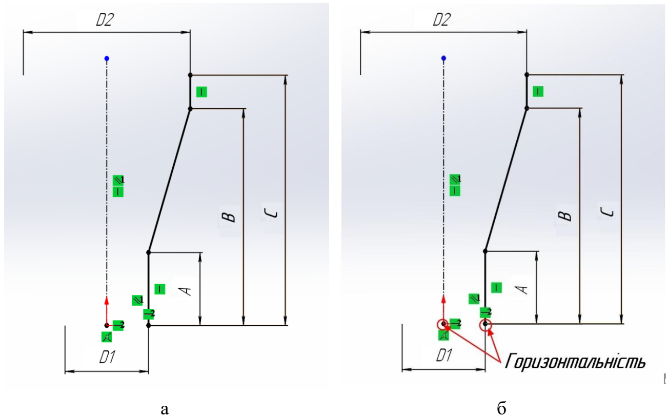
Рисунок 6.3 – Побудова ескізу, накладення взаємозв'язків
