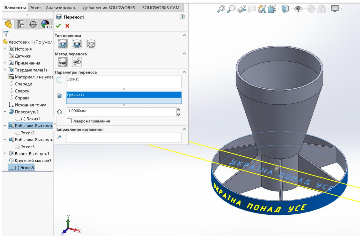
Рисунок 6.22 – Переміщення напису на поверхню деталі
