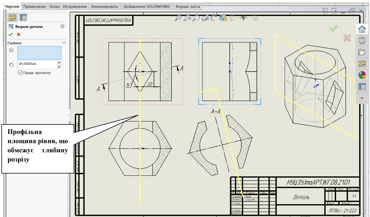
Рисунок 4.23 – Побудова профільного розрізу
