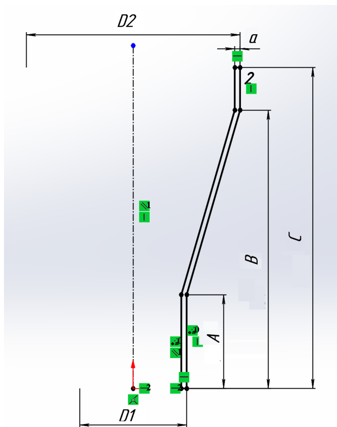
Рисунок 6.6 – Побудований ескіз контуру деталі
