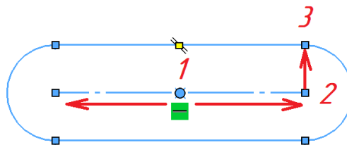
Рисунок 1.26 – Побудова прорізу через центральну точку
