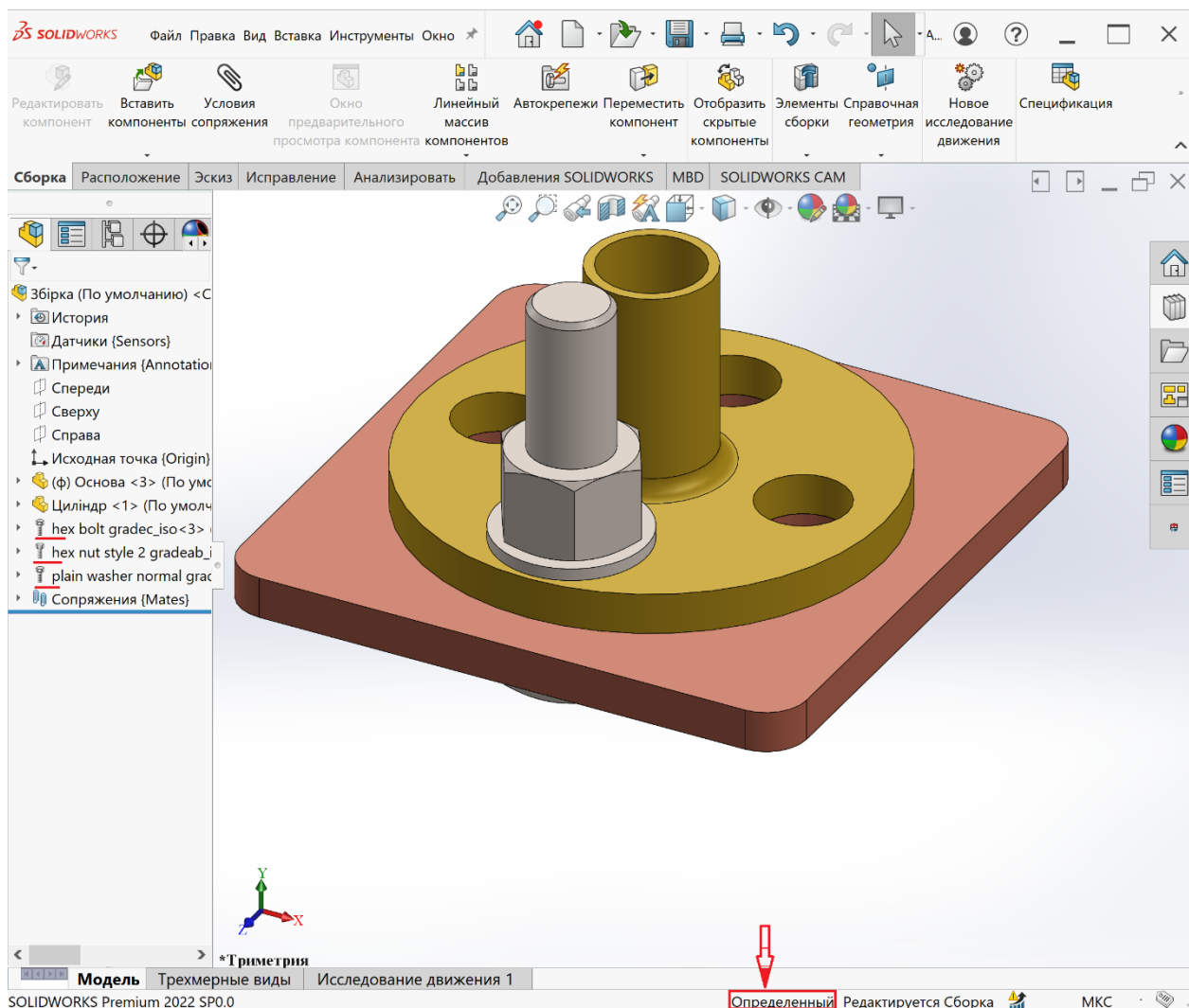
Рисунок 5.26 – З'єднання деталей за допомогою болтового з'єднання
