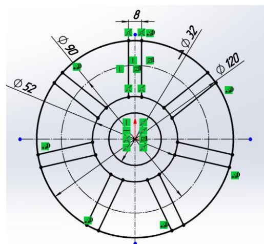
Рисунок 2.12 – Створений массив
