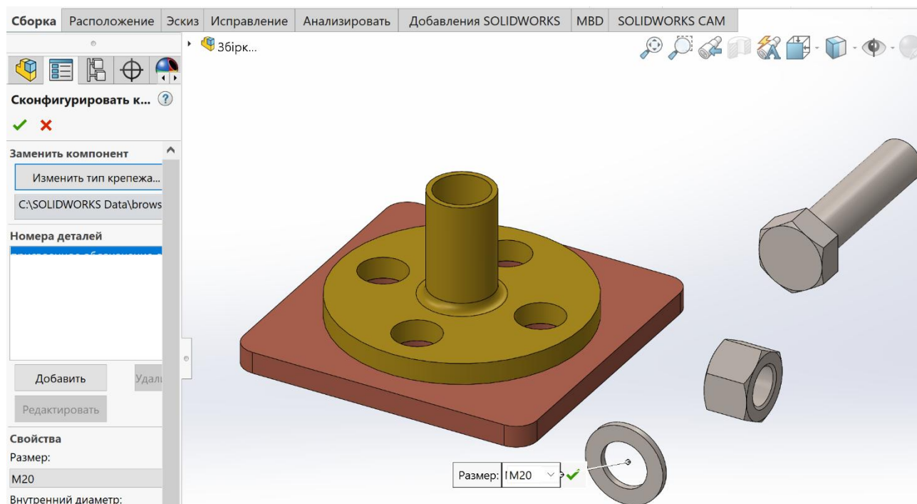
Рисунок 5.19 – Додавання шайби до збірки
