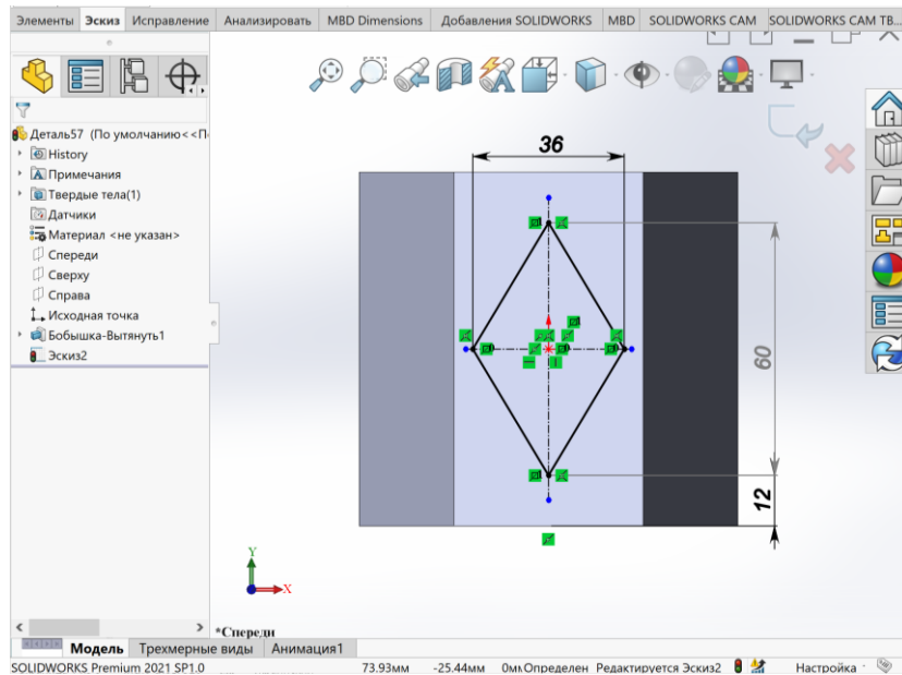
Рисунок 4.5 – Побудова ескізу отвору
