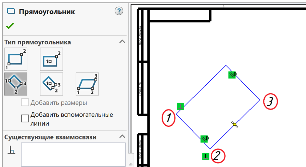
Рисунок 1.14 – Побудова прямокутника через 3 точки під кутом
