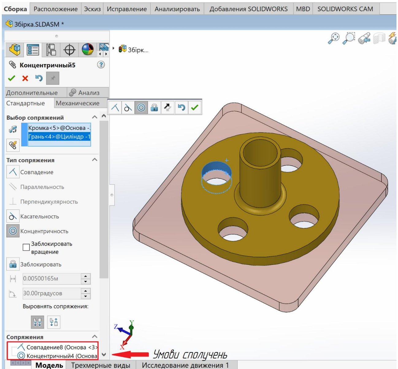
Рисунок 5.11 – Додавання умови Концентричність
