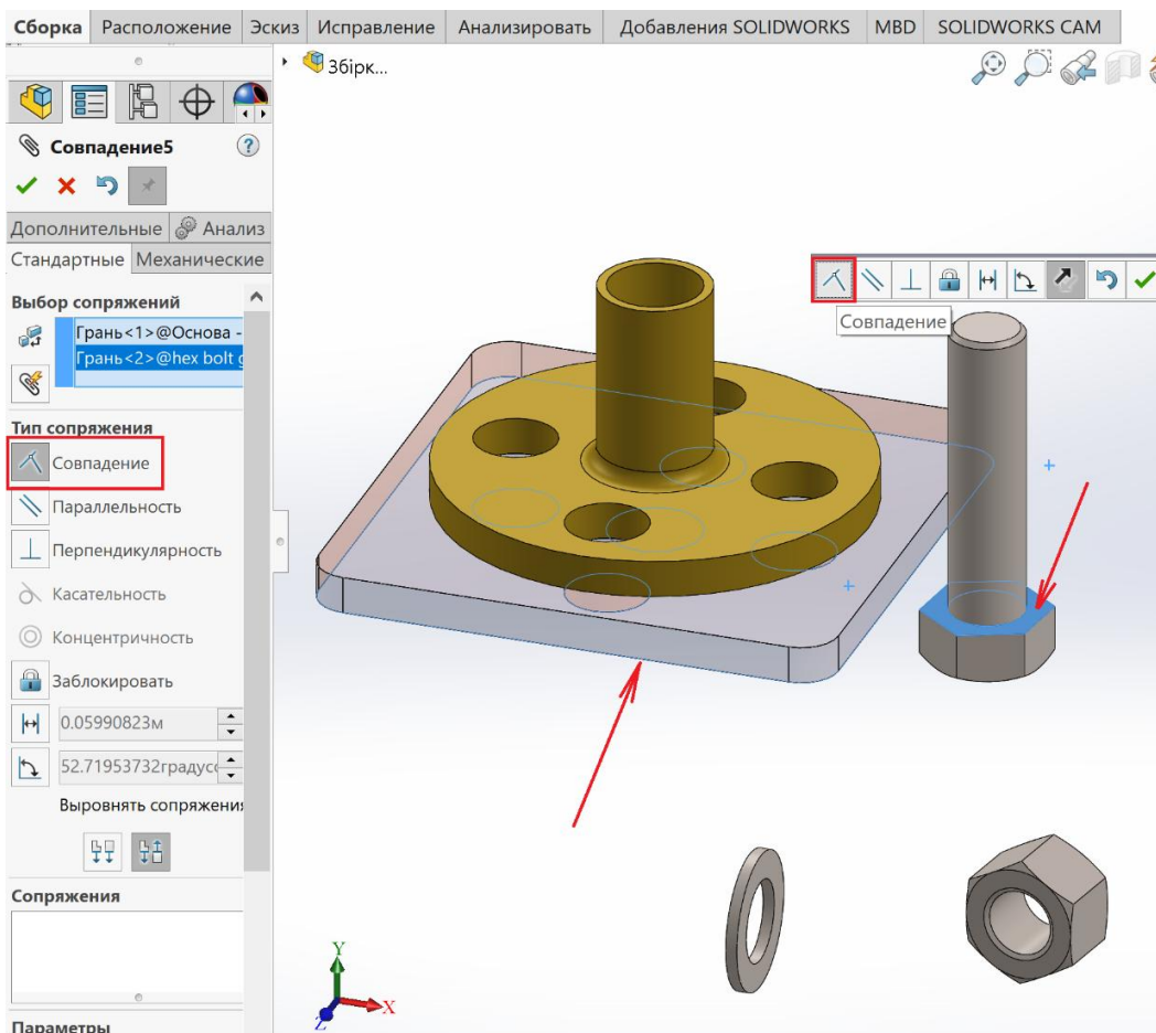
Рисунок 5.20 – Умова сполучення Збіг для основи та болта
