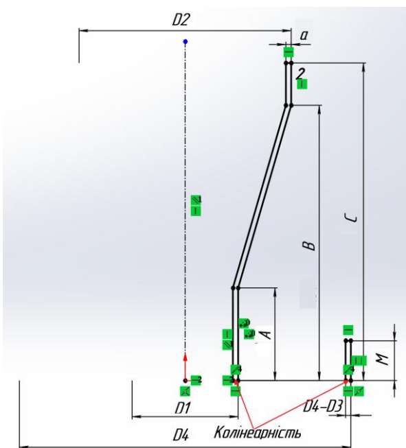
Рисунок 6.7 – Умова Колінеарність
