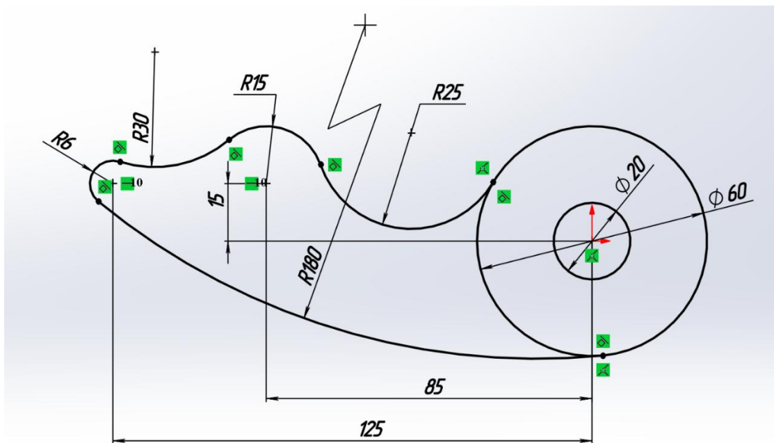
Рисунок 3.6 – Повністю визначений ескіз
