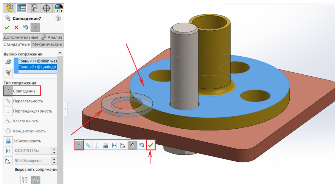
Рисунок 5.24 – Умова сполучення Збіг для шайби й циліндру
