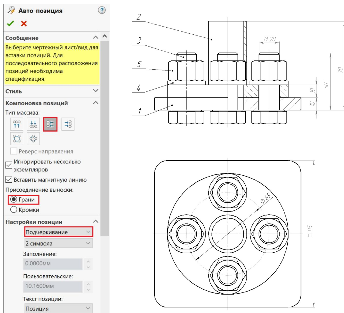
Рисунок 5.32 – Нанесення позицій для специфікації
