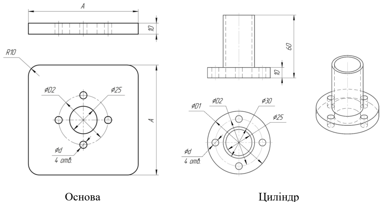
Рисунок 5.1 – Деталі для побудови збірки
