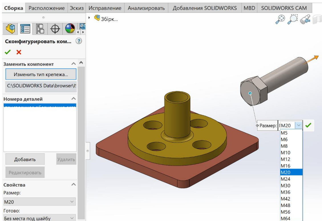
Рисунок 5.15 – Додавання болта до збірки
