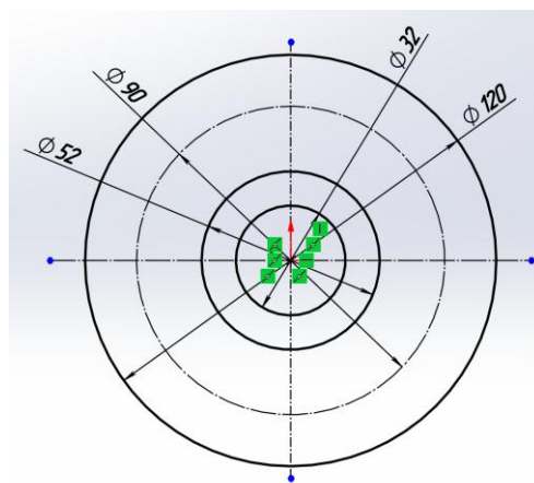
Рисунок 2.7 – Нанесення розмірів
