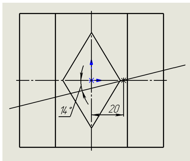
Рисунок 4.13 – Положення січної площини
