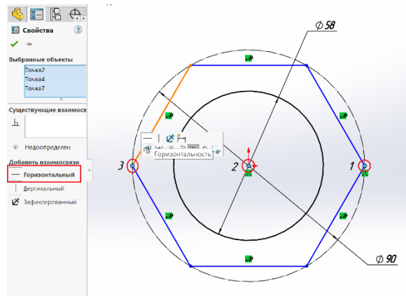
Рисунок 4.3 – Взаємозв'язки
