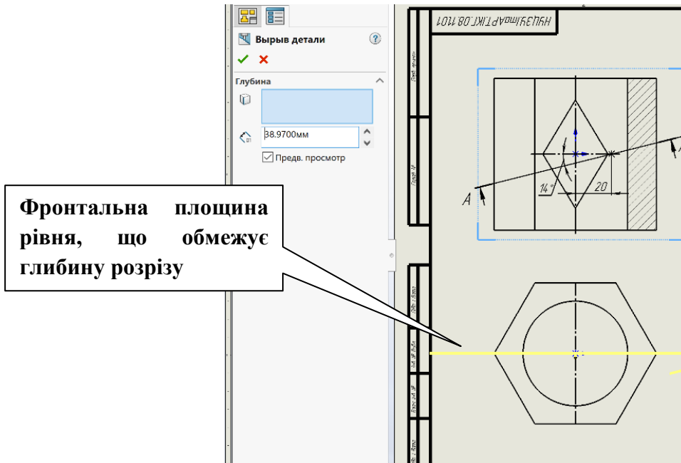
Рисунок 4.17 – Побудова фронтального розрізу
