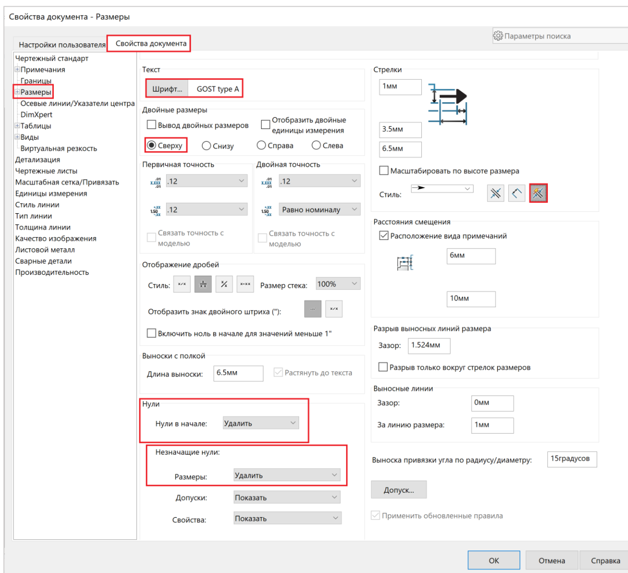
Рисунок 1.8 – Налаштування розмірів
