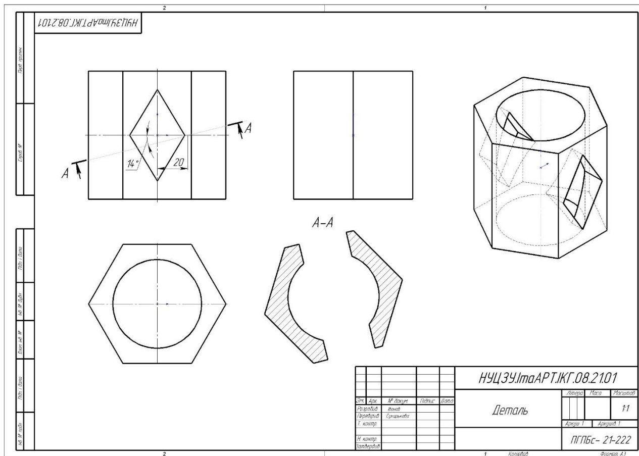
Рисунок 4.15 – Результат побудови перерізу
