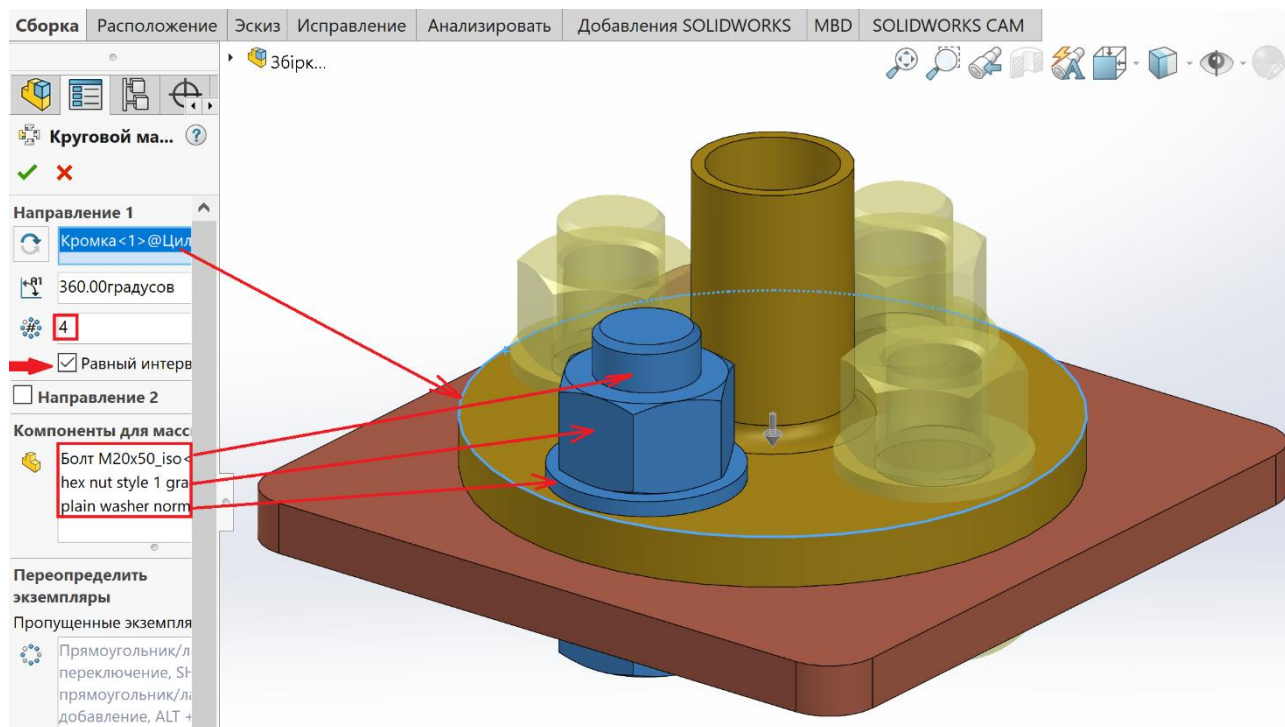
Рисунок 5.30 – Круговий масив болтового з'єднання
