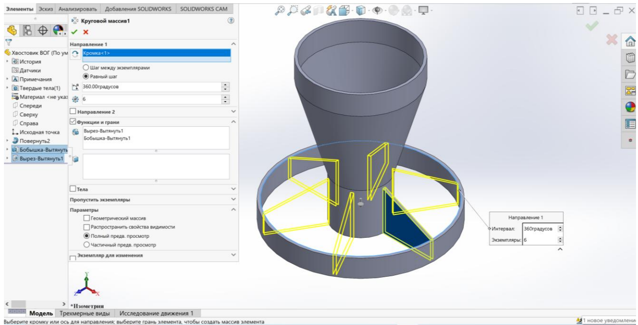
Рисунок 6.17 – Побудова кругового масиву елемента
