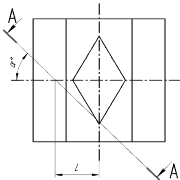
Рисунок 4.12 – Визначення розташування січної площини й кута нахилу
