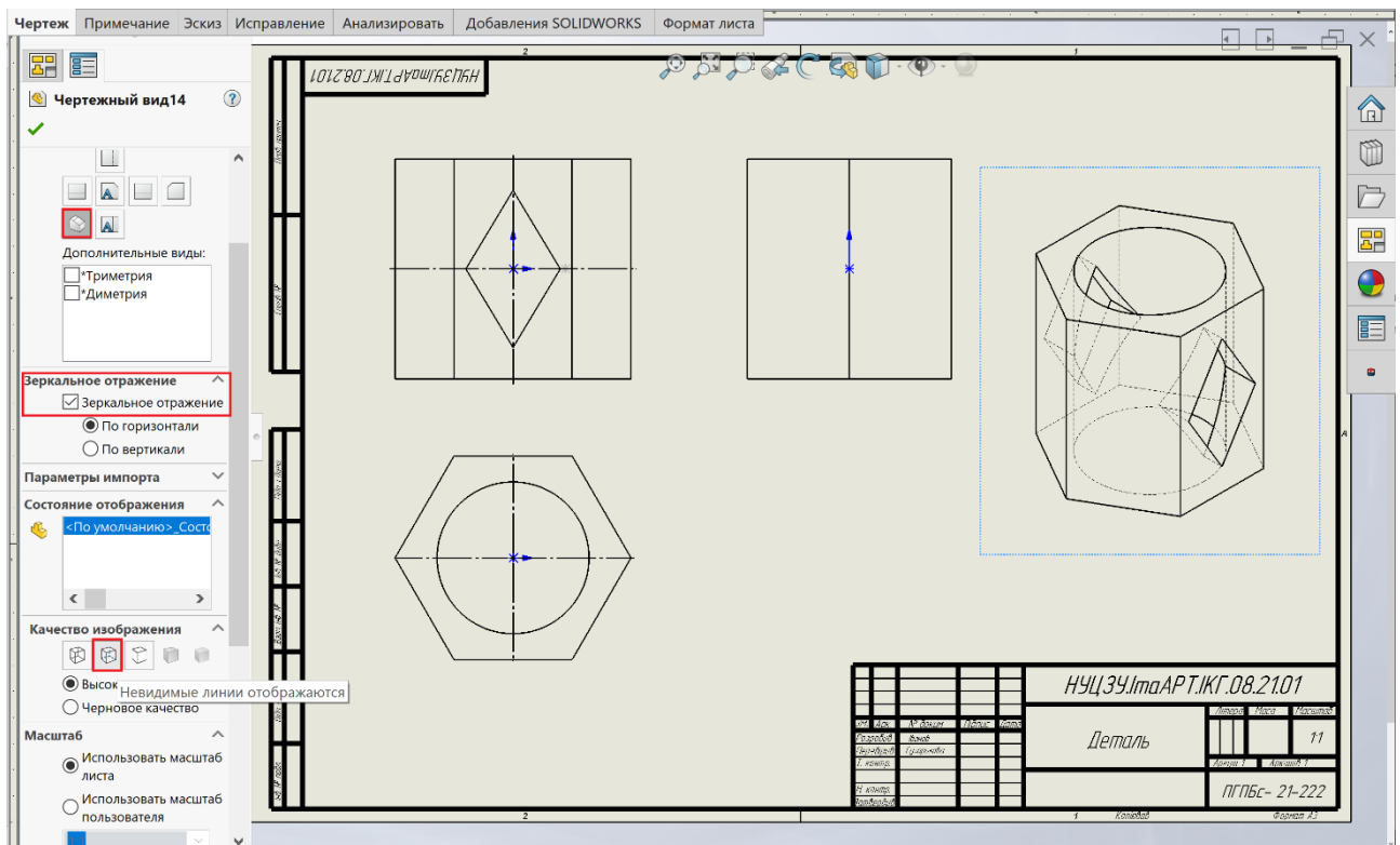
Рисунок 4.11 – Додавання на кресленик аксонометричного зображення
