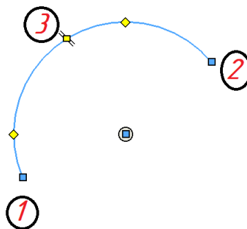
Рисунок 1.30 – Побудова дуги через три точки
