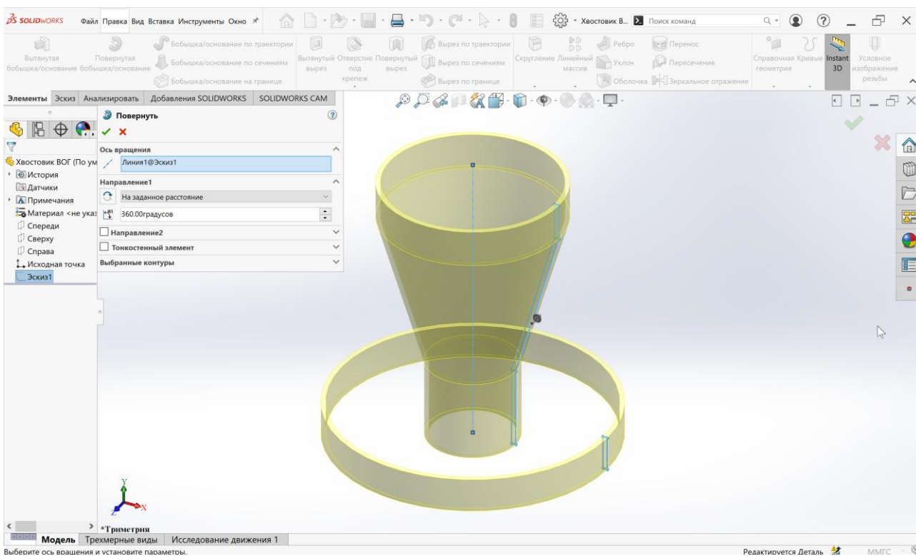
Рисунок 6.9 – Побудова елемента Повернена бобишка
