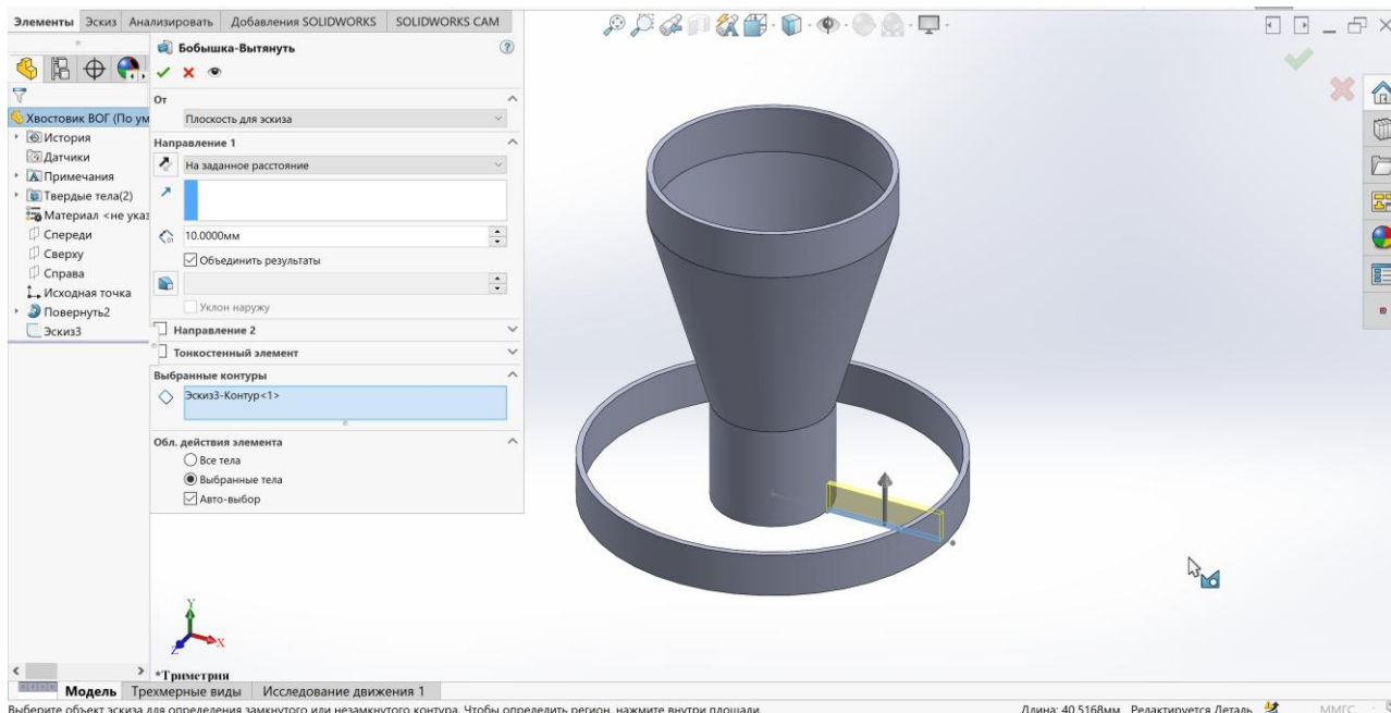
Рисунок 6.11 – Завдання параметрів для елемента Витягнута бобишка
