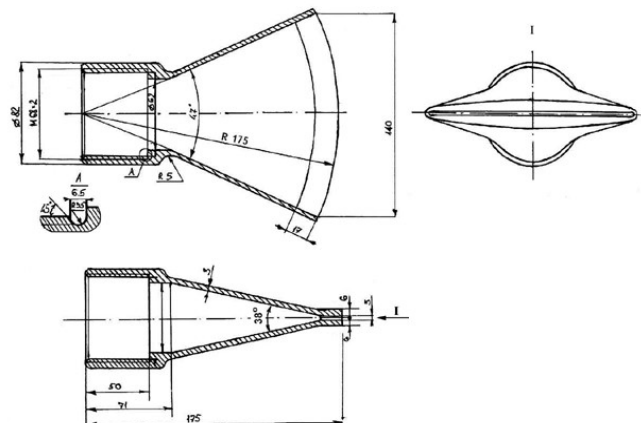
Рис. 1 – Загальний вигляд насадка для створення радіального водяного струменя
