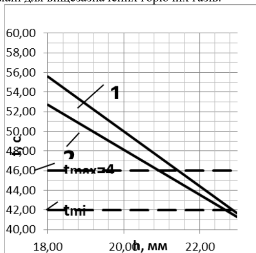
Рисунок 2 – Залежності часу підвищення температури мідного блоку в інтервалі від 100 °С до 700 °С від висоти полум'я, отримані для пальника потужністю 50 Вт при застосуванні метану (залежність 1) та пропан-бутану (залежність 2)
