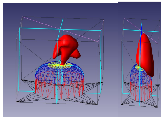
Ізоповерхня 1000°C
