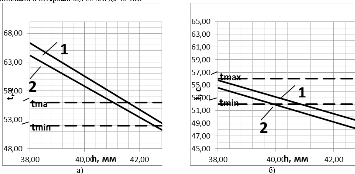
Рисунок 3 – Залежності часу підвищення температури мідного блоку в інтервалі від 98 °С до 703 °С (залежність 1) та від 102 °С до 697 °С (залежність 2) від висоти полум'я для пальника потужністю 500 Вт на газі метані (а) та на газі пропан-бутані (б)
