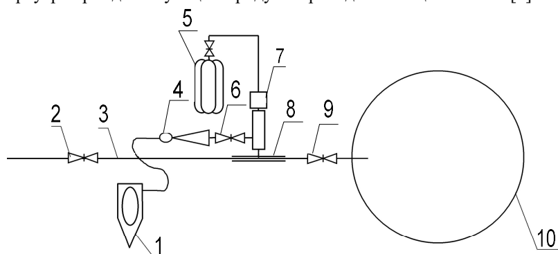
1 – пожарный аварийно-спасательный автомобиль; 2, 6, 9– шаровый кран (здвижка); 3 – действующий продуктопровод; 4 – высоконапорный генератор пены; 5 – источник сжатого воздуха; 7 – устройство врезки; 8 – бандаж; 10 – резервуар Рисунок 1 – Принципиальная схема реализации способа подачи воздушно-механической огнетушащей пены в резервуар через действующий продуктопровод
