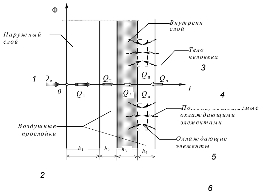
Рис. 1. Розрахункова схема оболонки
