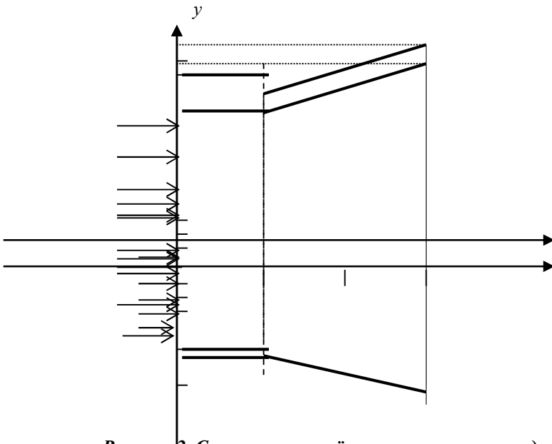
Рисунок 2. Схема проточної частини каналу насадка на пожежний лафетний ствол для створення плоскорадіального водяного струменя-екрана.
