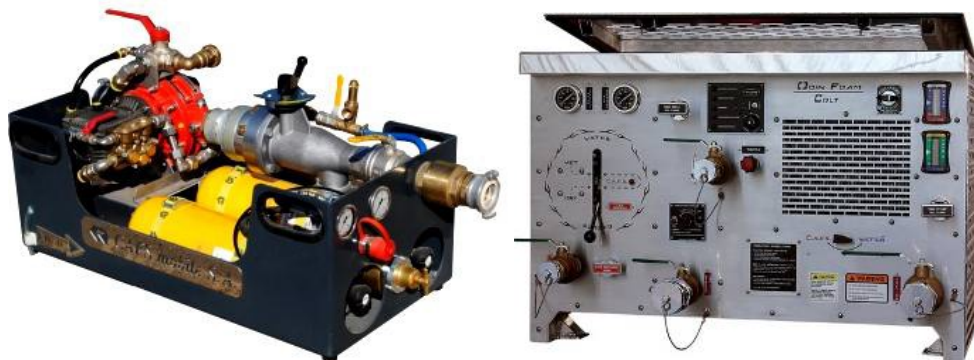
Рисунок 2 - Мобільна система («CAMS Mobile» Росія) та портативна система («CAMS 60-P» США)
