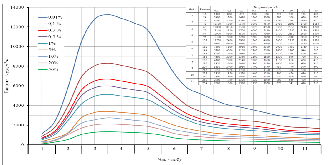
Рис. 1. Розрахункові гідрографи дощових паводків р. Дністер.
