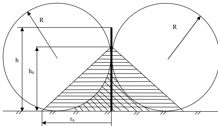
Рисунок 1 – Переріз у вертикальній площині зон захисту одиничного стрижньового блискавковідводу, розрахованих методом, що регламентується національним стандартом [4] та методом сфери, що котиться (стандарт ІЕС [9])
