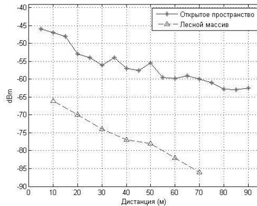
Рис. 5. График зависимости мощности сигнала от дистанции в различных средах
