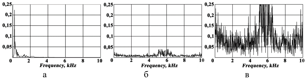
Рис. 2 – Результати моделювання – частотні спектрограми:
