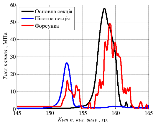
Рисунок 2 – Тиск палива у надплунже-рних порожнинах та в кармані розпи-лювача форсунки
