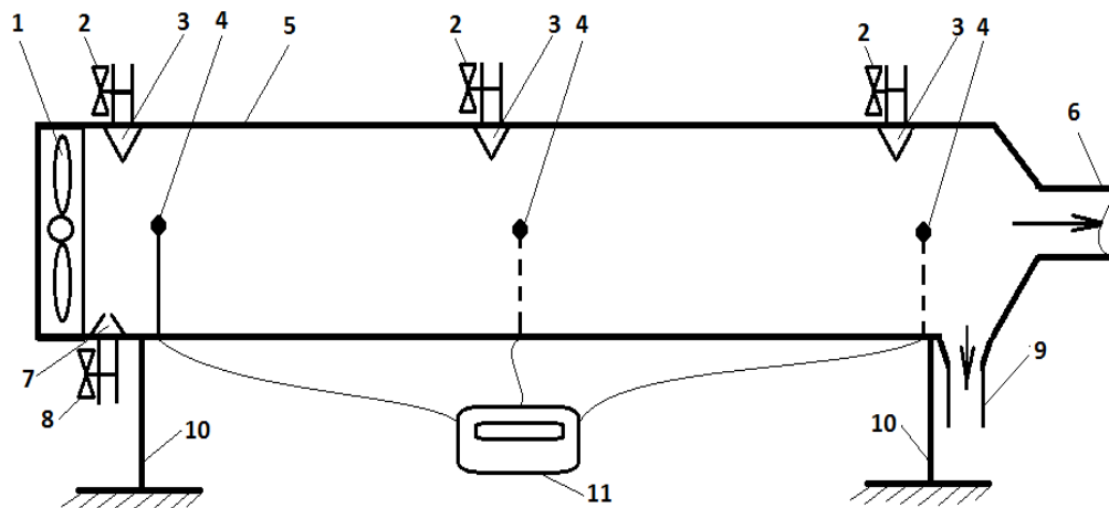
Рисунок 1 – Схема камери для дослідження процесів сорбції газів: 1 – вентилятор; 2 – рідинні запірні крани; 3 – рідинні форсунки; 4 – газоаналізатори; 5 – корпус; 6 – відвідний газовий патрубок; 7 – газова форсунка; 8 – газовий запірний кран; 9 – відвідний рідинний патрубок; 10 – кріплення; 11 – блок індикації газоаналізаторів.
