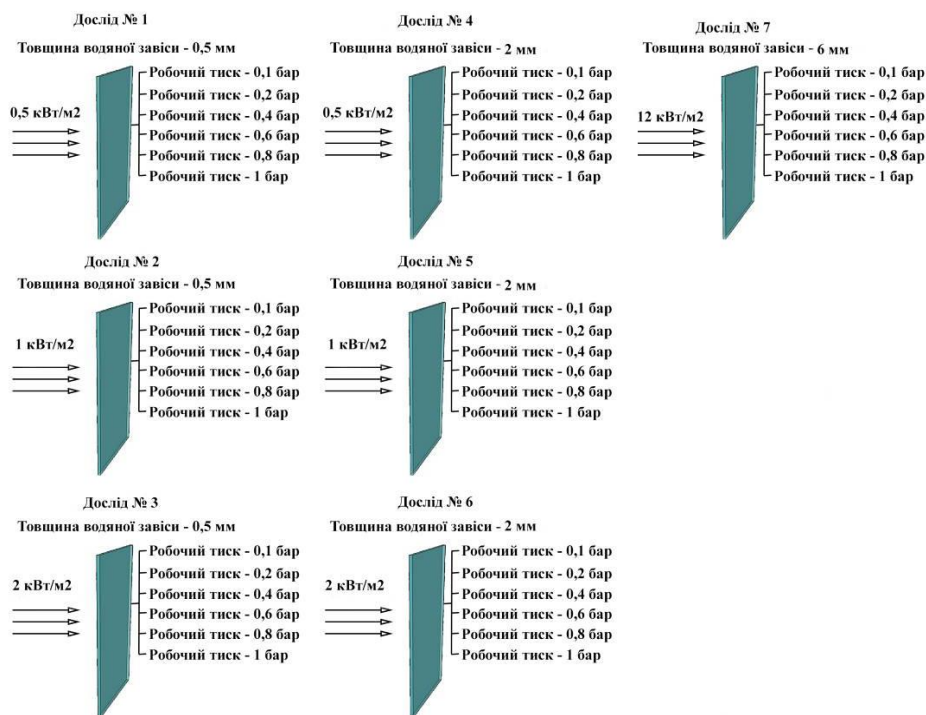
Рисунок 2 – Схема послідовності проведення експериментальних досліджень.
