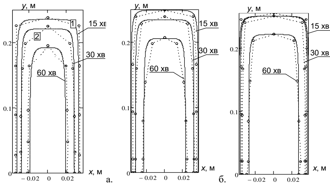
Рис. 1. Розташування лінії контуру зони обуглювання, апроксимованої за допомогою кривої Без'є у перерізі дерев'яної балки 70×250 без вогнезахисту (а), із вогнезахисним облицюванням w = 10 мм (б); із вогнезахисним облицюванням w = 20 мм (в) у різні моменти часу впливу стандартного температурного режиму пожежі: 1 – розрахункові дані; 2 – експериментальні дані.
