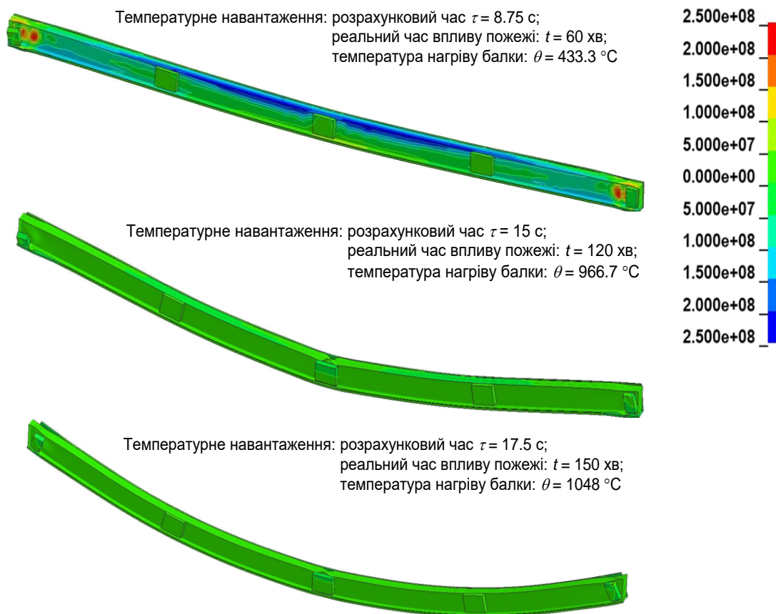
Рис. 2 Розподіл поздовжніх нормальних напружень на різних етапах прикладення температурного навантаження
