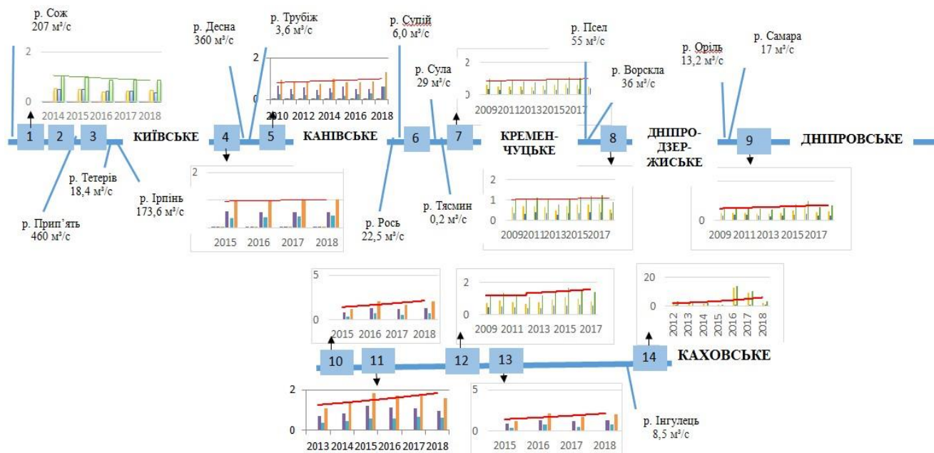
Рисунок – 2 Схема формування водотоку басейну Дніпра, з позначенням основних 15 приток та відображення їх витрат води, а також графічним відображенням змін сумарного вмісту аніонів
