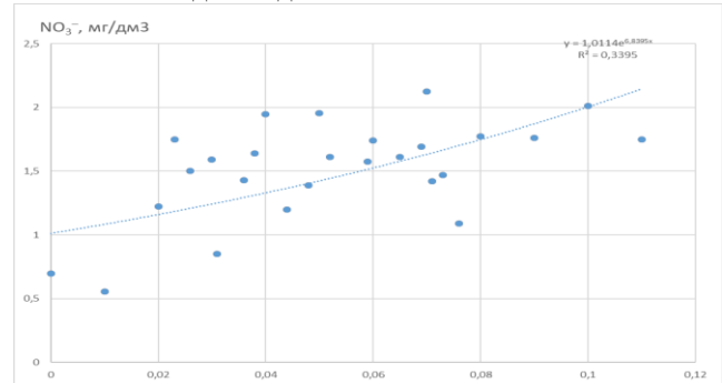
Рисунок – 7 Кореляційна залежність між середньорічними концентраціями нітрит та нітрат іонів в воді Дніпра за період 2009-2018 рр.
