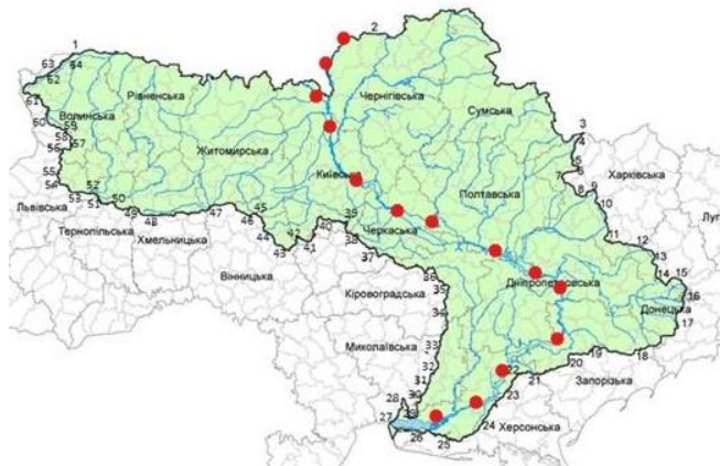
Рисунок – 1 Схематичне розміщення 14 постів контрольного забору води, за даними яких проводилось дослідження
