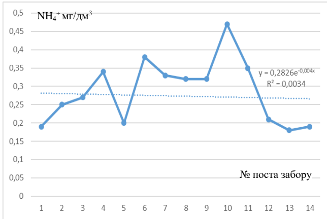
Рисунок – 5 Загальний вміст амонію NH 4 + по постах заборів води басейну Дніпра за 2017 рік.
