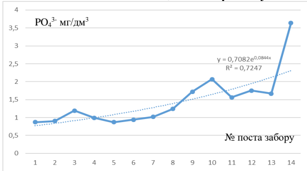
Рисунок – 3 Загальний вміст аніонів по постах заборів води басейну Дніпра за 2017 рік.
