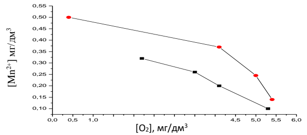
Рисунок – 10 Залежність концентрації іону мангану від концентрації розчиненого кисню у воді водосховища.
