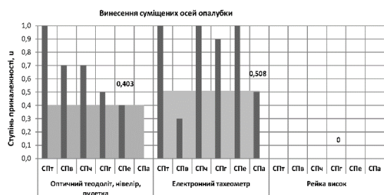
Рис. 2. Ступінь впливу факторів при винесенні суміжних осей положення опалубки колон
