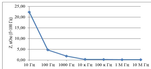
Рис. 2. Полное электрическое сопротивление системы Z РЖ
